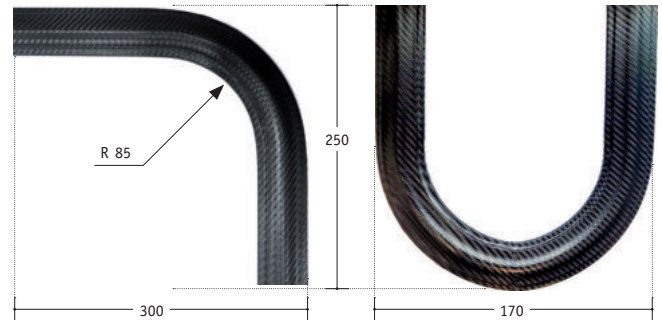
Handlauf-Winkelelement
