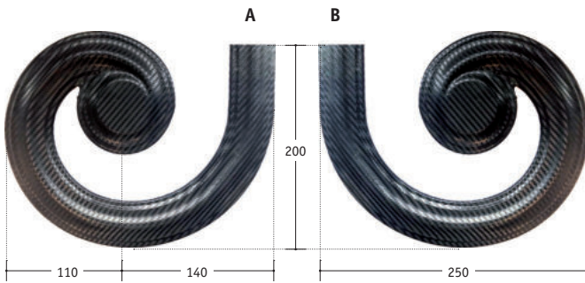
Handlauf-Anfangsstück
